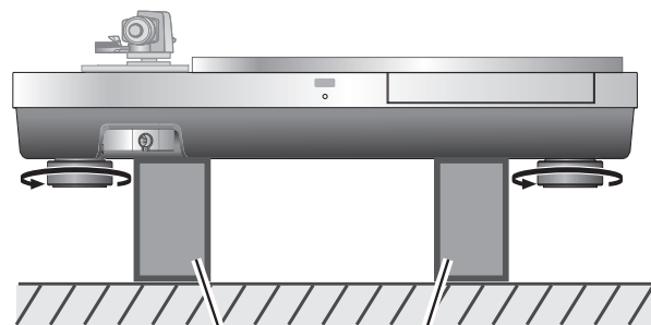
Coussin d'emballage
