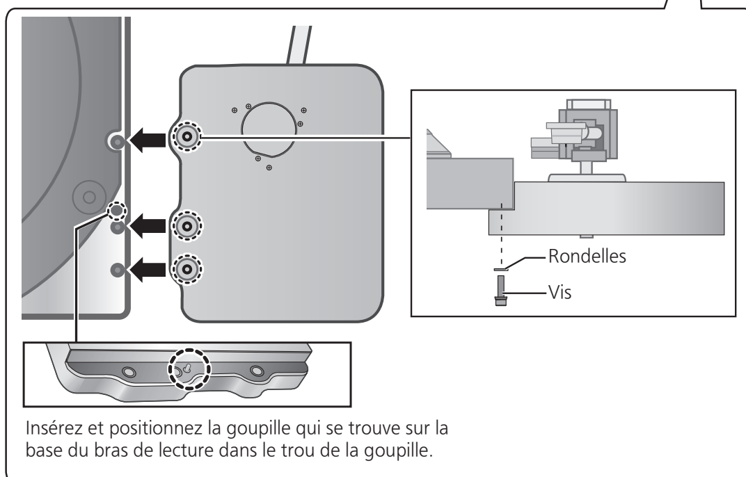
Position standard pour le montage de la base du bras de lecture
