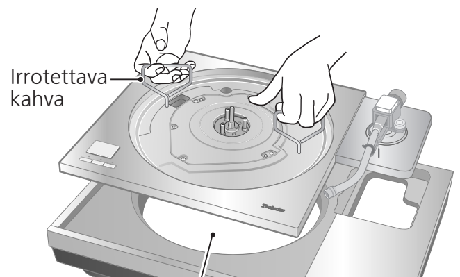
Pujota ohjausyksikön liitäntäjohto levylautasen jalustan läpi.
