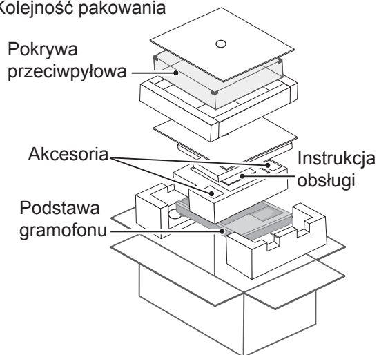
Kolejność pakowania
