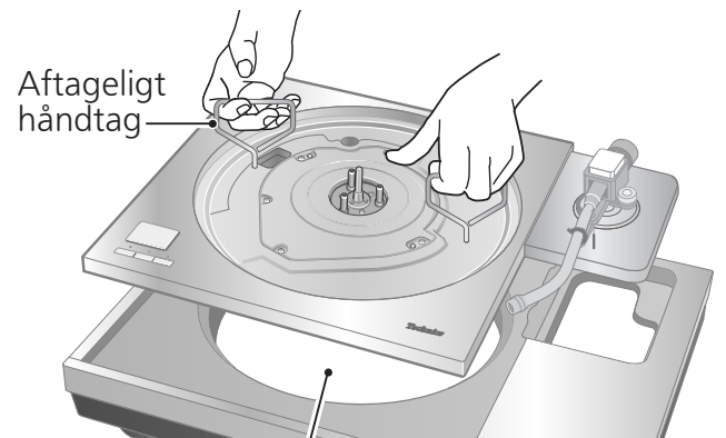
Før stikket til tilslutning af styreenhed ind gennem hullet på pladetallerkenens base.
