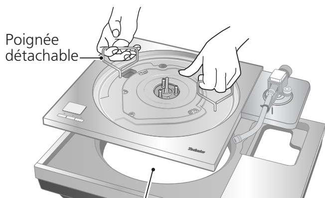
Trou de montage de la poignée détachable
