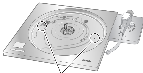
Trous de montage des poignées détachables
