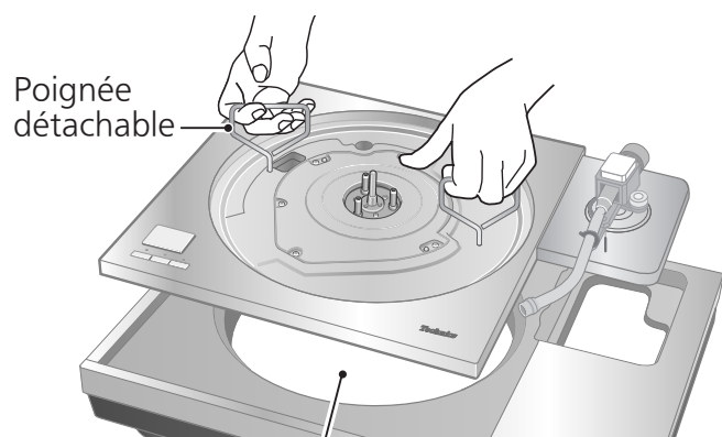
Trous de montage des poignées détachables
